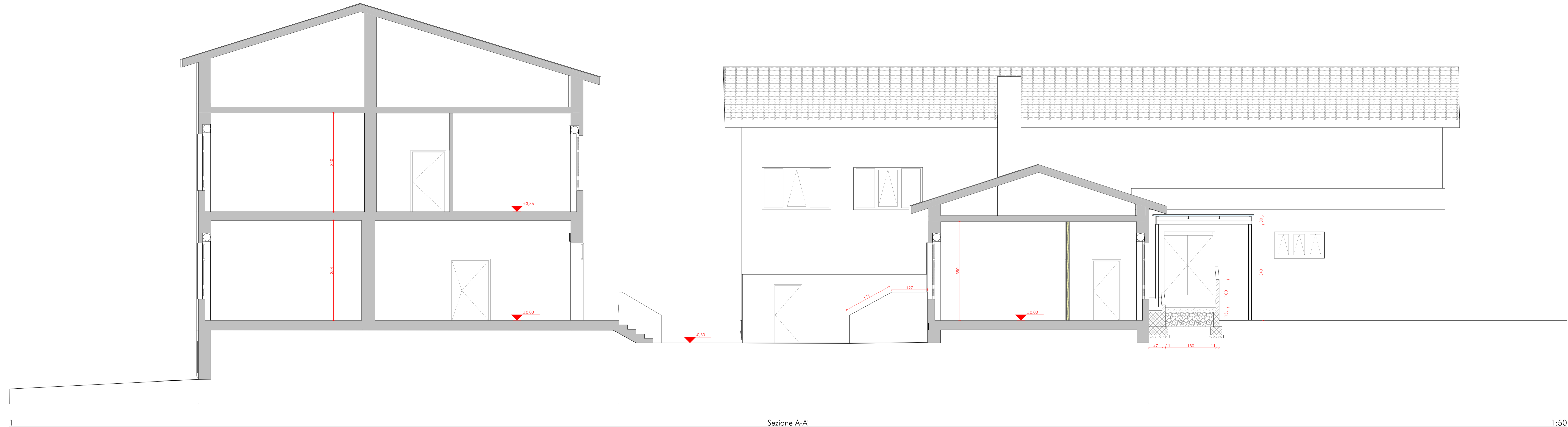
Sezione A-A'
