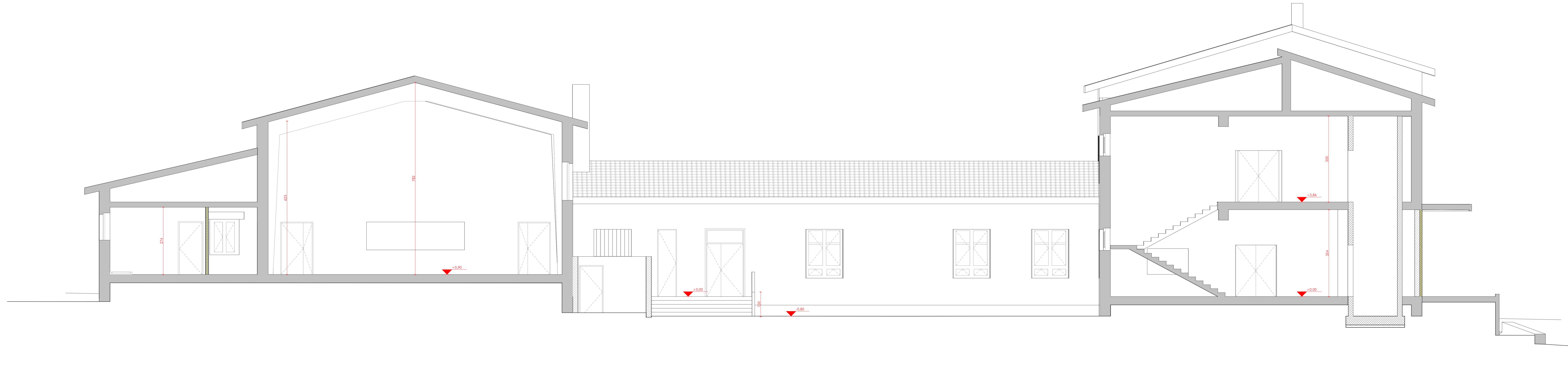
Sezione B-B1
