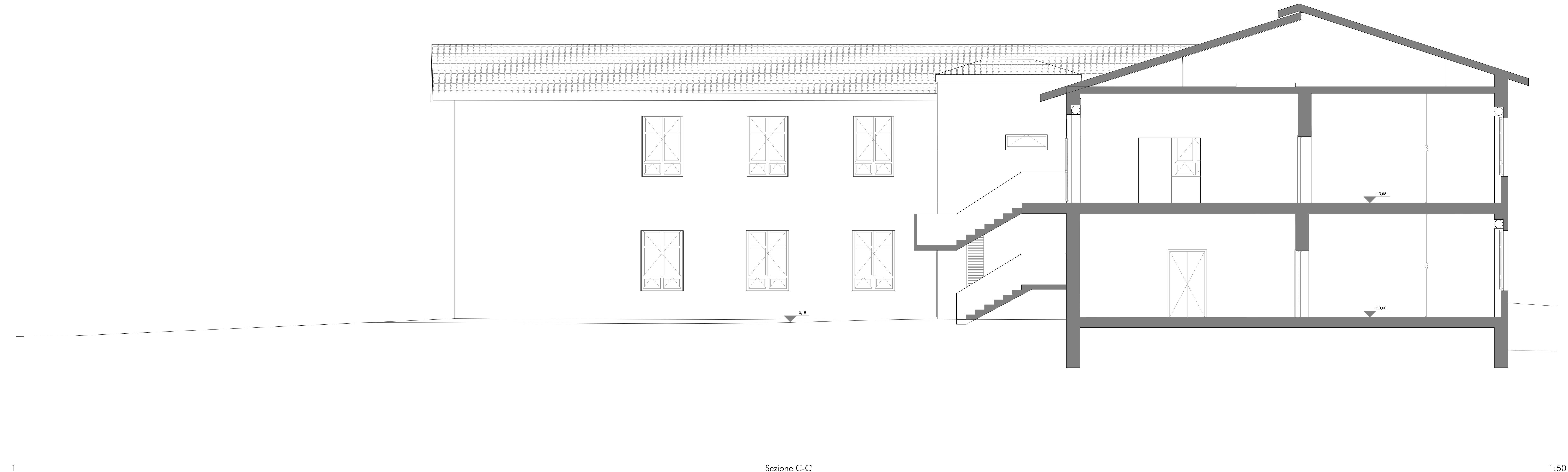
Sezione C-C'
